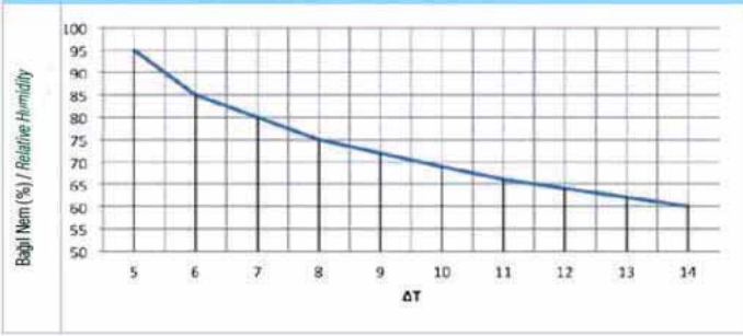
Oda bağıl neminin \Delta T sıcaklık farkına göre değişimi Change of relative humidity in ambient in regard to \Delta T
